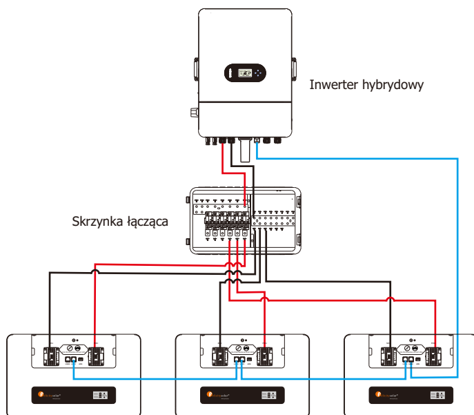
Rysunek 4-1 Połączenie równoległe trzech zestawów akumulatorów
