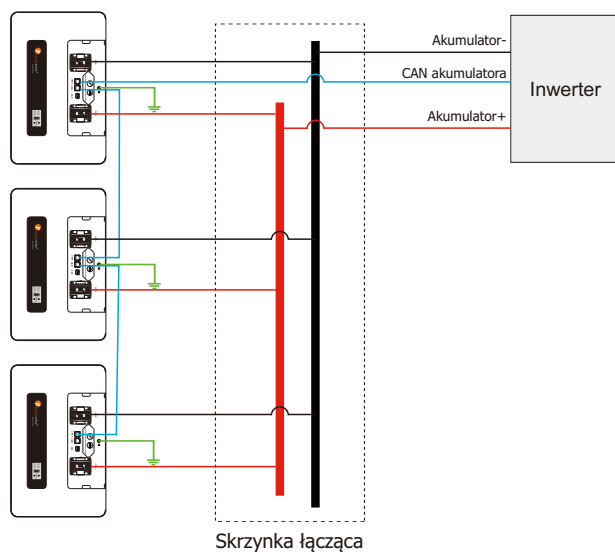
Rysunek 4-1 Połączenie równoległe trzech zestawów akumulatorów
